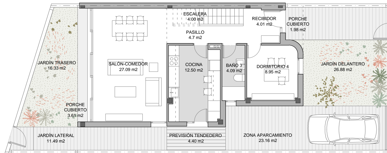
PLANTA BAJA
