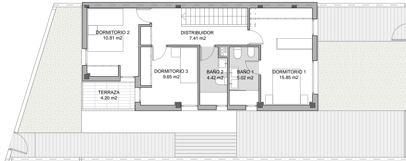
PLANTA PRIMERA
